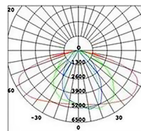
Fotometria media-ampia
